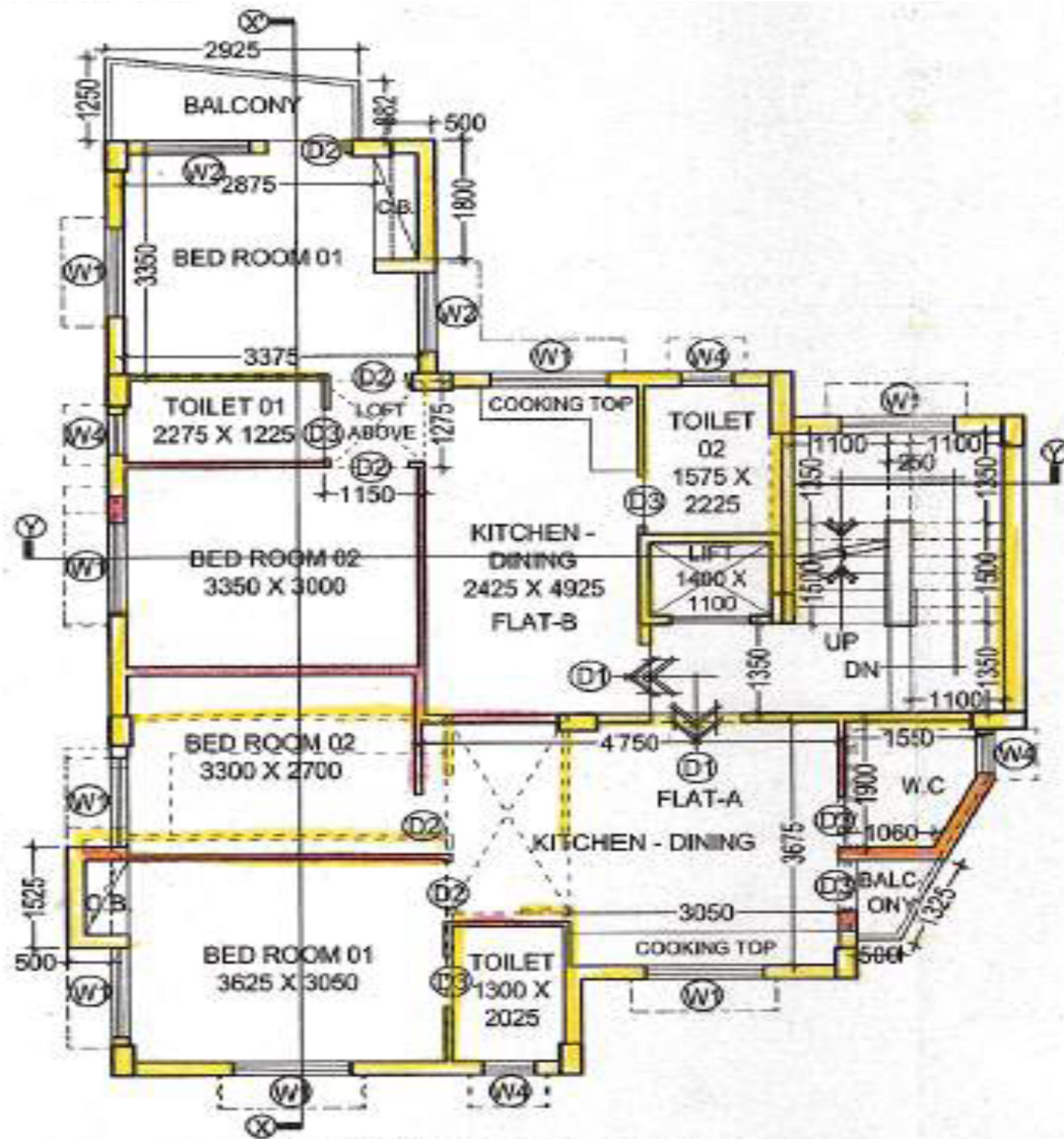
3rd. FLOOR PLAN. SCALE : 1 : 100
